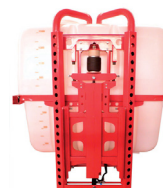
Elevación Hidráulica + Suspensión neumática
